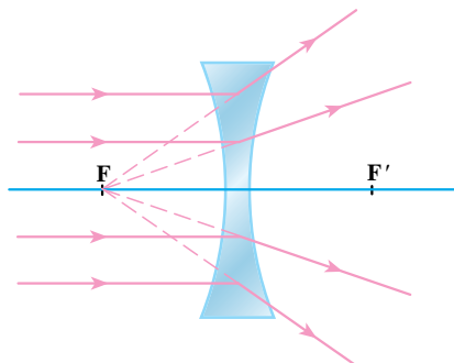
شکل ۲۸-۵- در عدسی واگرا پرتوهای تابش موازی محور اصلی باشند، پس از شکست عدسی و عبور از آن، طوری از هم دور می‌شوند که امتدادشان در یک نقطه همدیگر را قطع می‌کند.
